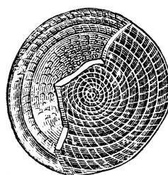
Nummulitesz
