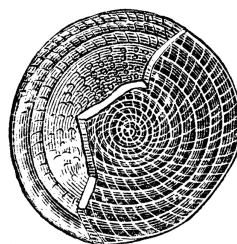
Nummulitesz
