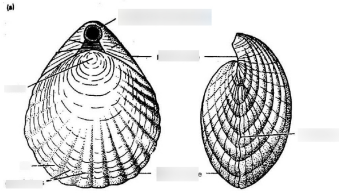
Brachiopoda/pörgekarú
