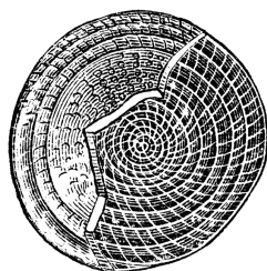
Nummulitesz
