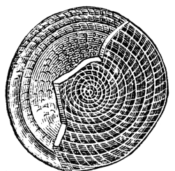
Nummulitesz
