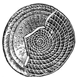
Nummulitesz
