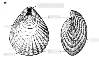
Brachiopoda/pörgekarú
