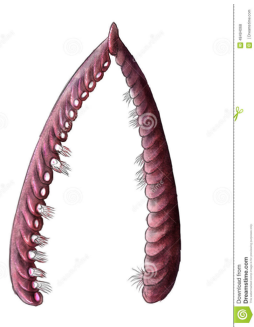
Graptolit
