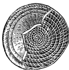
Nummulitesz
