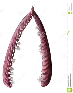
Graptolit
